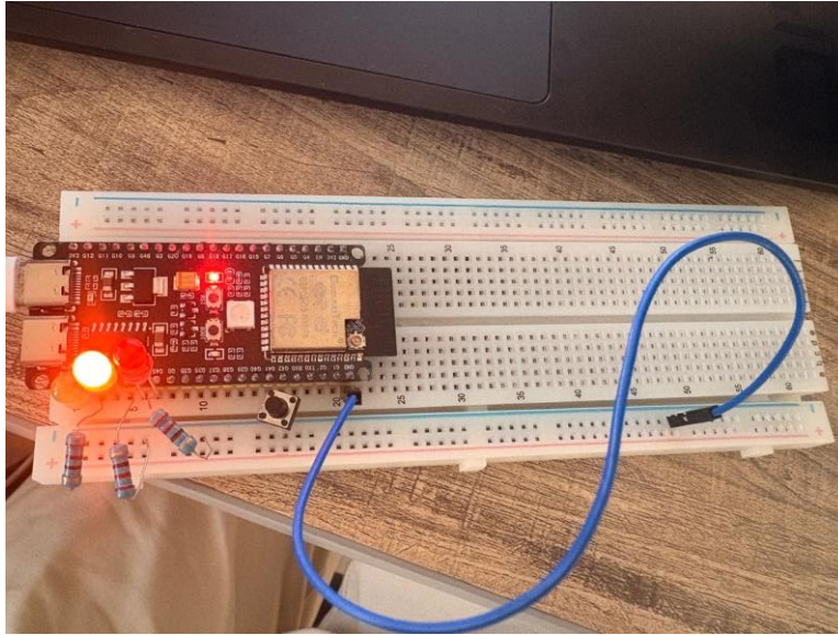
Ilustración 12 Semáforo inteligente "En naranja"
