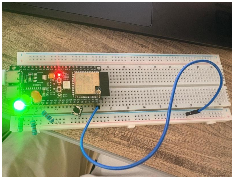
Ilustración 13 Semáforo inteligente "En verde"
