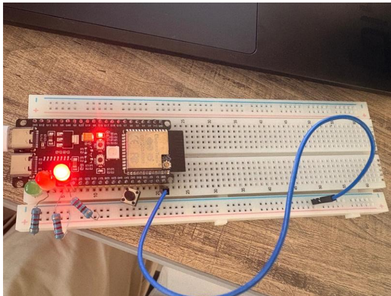
Ilustración 11 Semáforo inteligente "En rojo"
